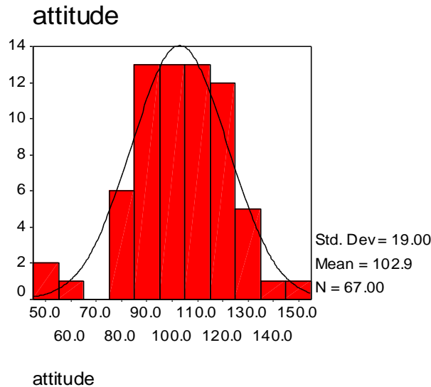
نمودار ۲- توزیع نرمال نمره‌های نگرش به درس مبانی جامعه‌شناسی دانشجویان دختر
