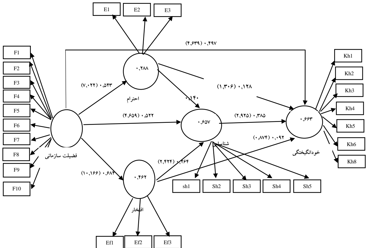
شکل ۲- مقادیر R^2 و الگوی ساختاری
